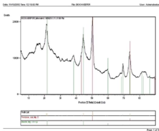
Fot. 17. Analiza składu odparowanej próbki preparatu Bookkeeper metodą mikrodyfrakcji rentgenowskiej (XRD). Stwierdzono obecność tlenku magnezu – MgO i wodorotlenku magnezu – Mg(OH) 2
