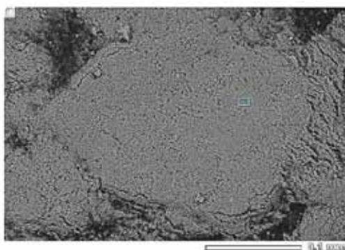
Fot. 18. Analiza składu pierwiastkowego odparowanej próbki preparatu Bookkeeper. Stwierdzono obecność następujących pierwiastków: Mg, O, C, F. Fluor pochodzi z przypuszczalnie z surfaktantu stanowiącego jeden ze składników preparatu
