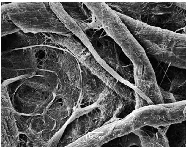
Fot. 7. Czysta bibuła Whatman jest materiałem o dużej mikroporowatości. Widoczne są włókna roślinne poddane procesowi fibrylacji podczas produkcji. Obraz SEM-SE
