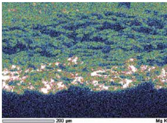
Fot. 11. Mapowanie przeprowadzone na przekroju czystej bibuły Whatman, po odkwaszeniu, przed starzeniem (widoczny ten sam fragment próbki, co na fot. 10)
