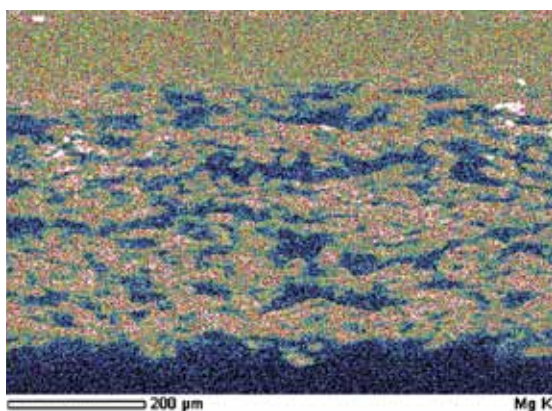
Fot. 13. Mapowanie przeprowadzone na przekroju próbki testowej z farbą olejną po odkwaszeniu i przyspieszonym starzeniu klimatycznym (widoczny ten sam fragment próbki, co na fot. 12). Związki magnezu rozłożone są równomiernie. Niewielkie zwiększenie ich koncentracji można zaobserwować w pobliżu warstwy farby
