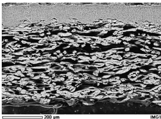
Fot. 12. Przekrój próbki testowej z farbą olejną po odkwaszeniu i przyspieszonym starzeniu klimatycznym. Cząstki preparatu w dolnej części próbki nie są zauważalne na obrazie SEM. Obraz SEM-BSE
